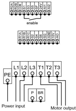
Schaltplan:
