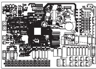
Indoorprintplaat
