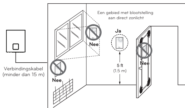
Draadloze luchttemperatuursensor
