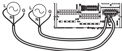
1Ø reserveverwarming (Voor Split R32 Binneneenheid 4-serie)
