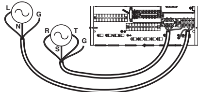
3Ø reserveverwarming (Voor Split R410A Binneneenheid 3-serie)
