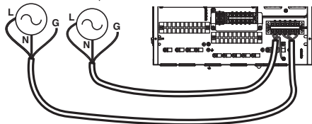
1Ø reserveverwarming (Voor Split R410A Binneneenheid 3-serie)
