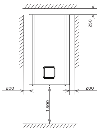
Minimale serviceruimte (Eenheid : mm)
