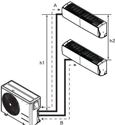
Mehrfach-Rohrleitungen
