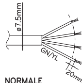
NORMALE DWARSDOORSNEDE GEBIED 0.75mm 2 H07RN-F
