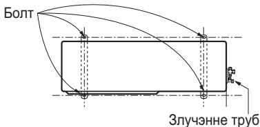
Злучэнне труб
