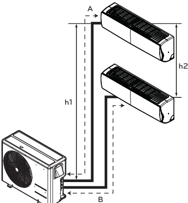
Mehrfach-Rohrleitungen
