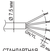
СТАНДАРТНАЯ ПЛОШЧА ПАПЯРОЧНАГА СЯЧЭННЯ 0.75 мм 2 H07RN-F
